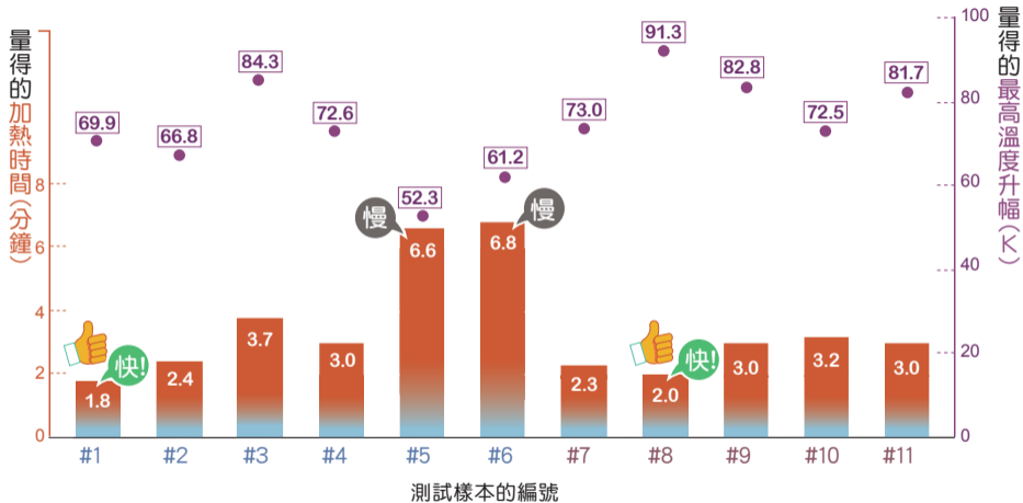
圖一：無葉風扇樣本暖風功能的加熱表現
