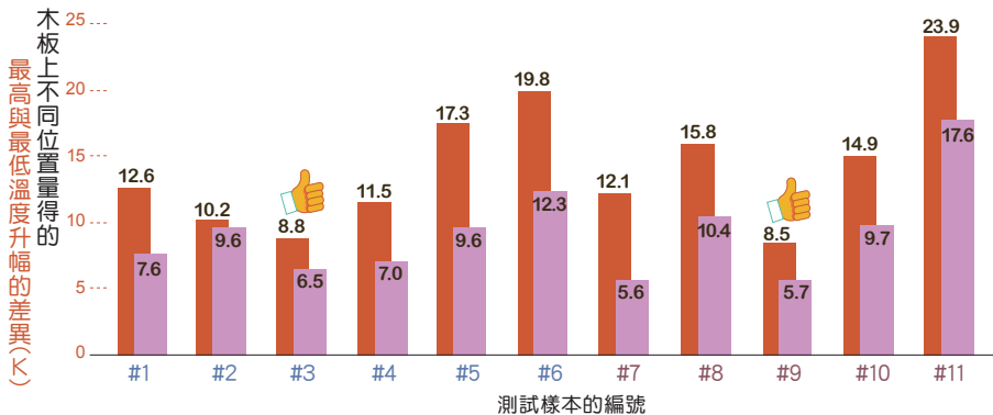
圖二：無葉風扇樣本暖風功能的熱力均勻度
