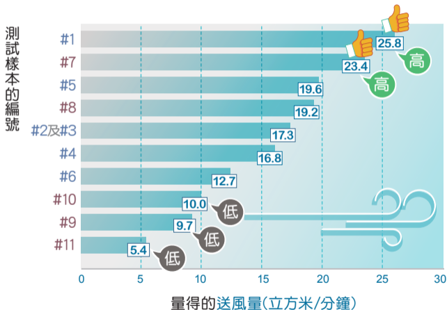
圖三：無葉風扇樣本涼風功能的送風表現
